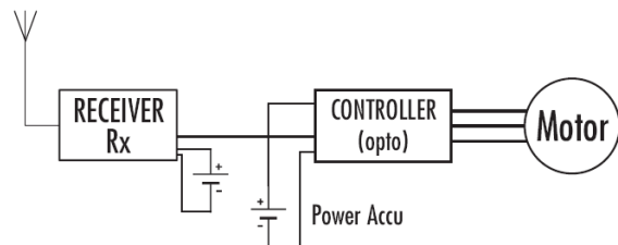
Schaltplan der Optoversion des Controllers (ohne BEC)
