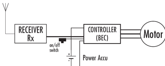
Schaltplan des Controllers mit BEC
